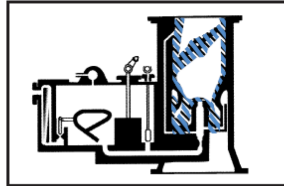
Carburetor icing
